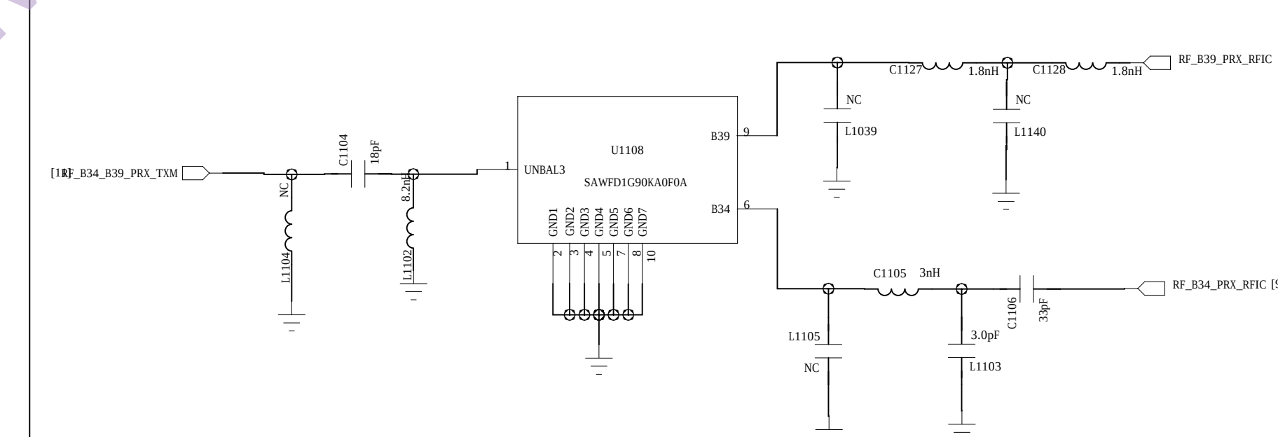
B34/39 PRX
